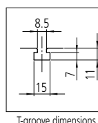
T-groove dimensions
